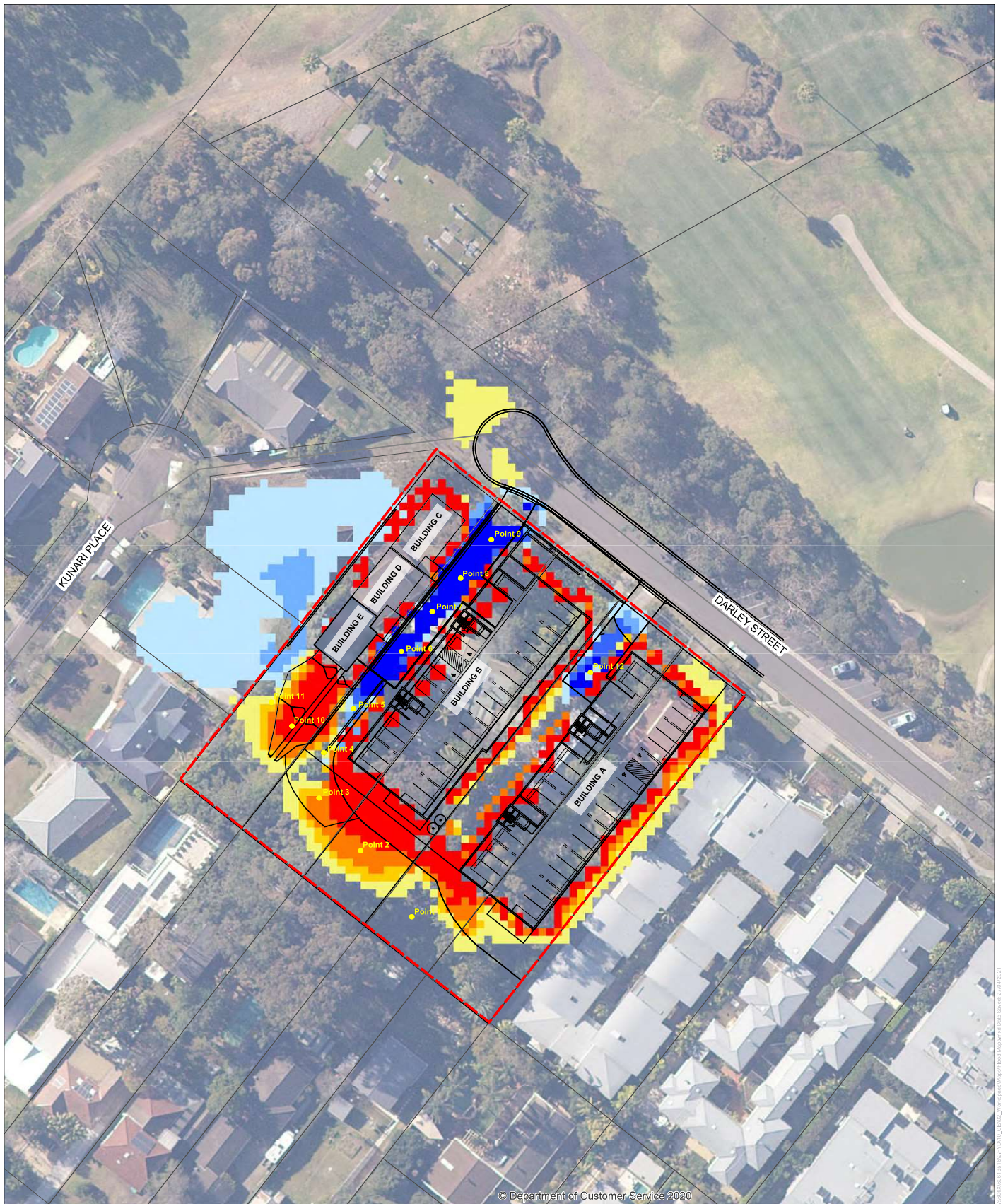
FIGURE 7: AFFLUX (PMF 15 MIN, D04-E01)
